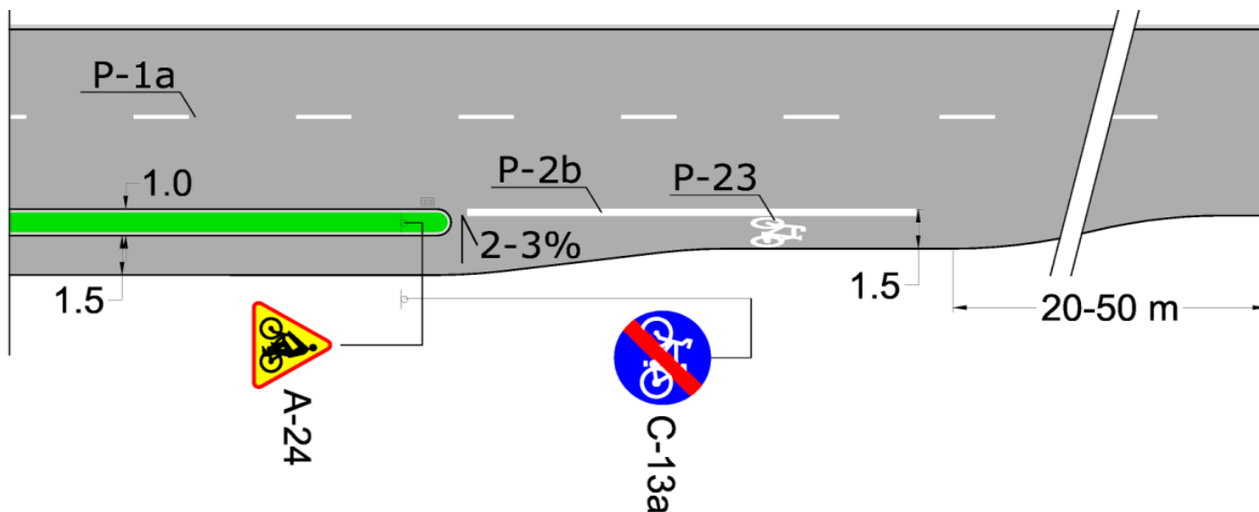
Rys. 17C. Koniec jednokierunkowej drogi dla rowerów
