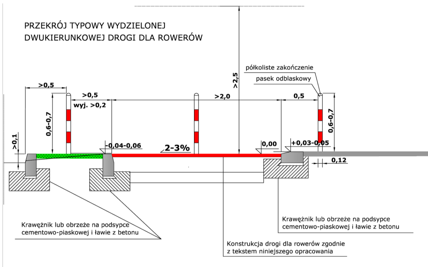
Rys. 13A. Zasady lokalizacji słupków blokujących U-12c w przekroju dwukierunkowej drogi dla rowerów. Jeden słupek musi znajdować się symetrycznie w osi drogi dla rowerów. Od jezdni dodatkowo drogę dla rowerów może oddzielać bariera ochronna U-14a. W przekroju zaznaczono dodatkowo skos zjazdu indywidualnego (słupki blokujące stosuje się m. in. w rejonie zjazdów, którymi samochody mogą nielegalnie wjeżdżać na drogę dla rowerów).
