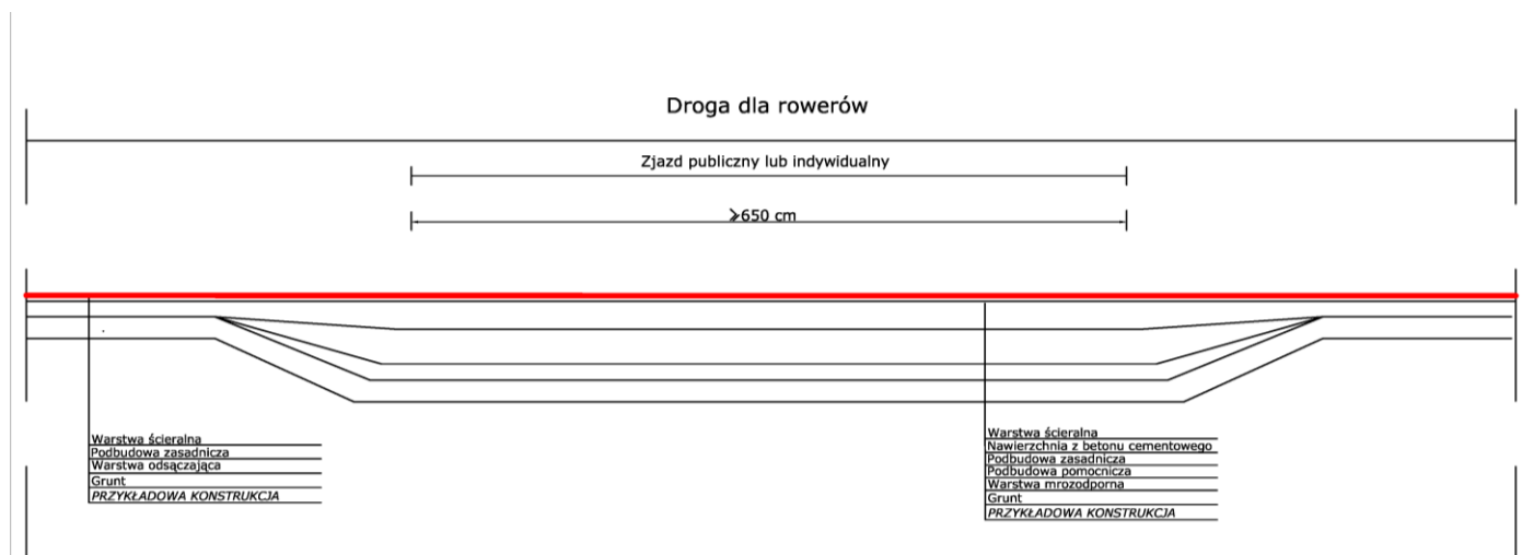
Rys. 12I. Przykład konstrukcji zjazdu publicznego lub indywidualnego – konstrukcja zjazdu nie jest ograniczona krawężnikami.
