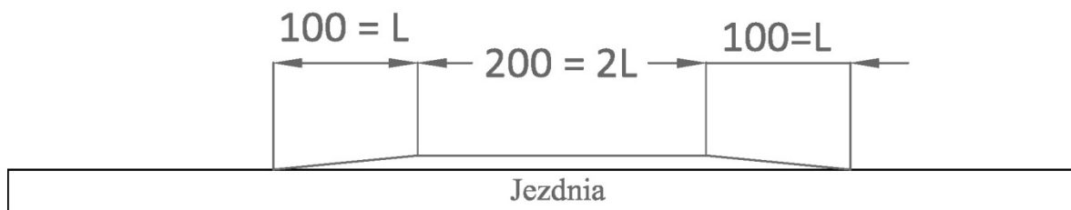
Rys. 1. Płytowy próg zwalniający – przekrój podłużny
