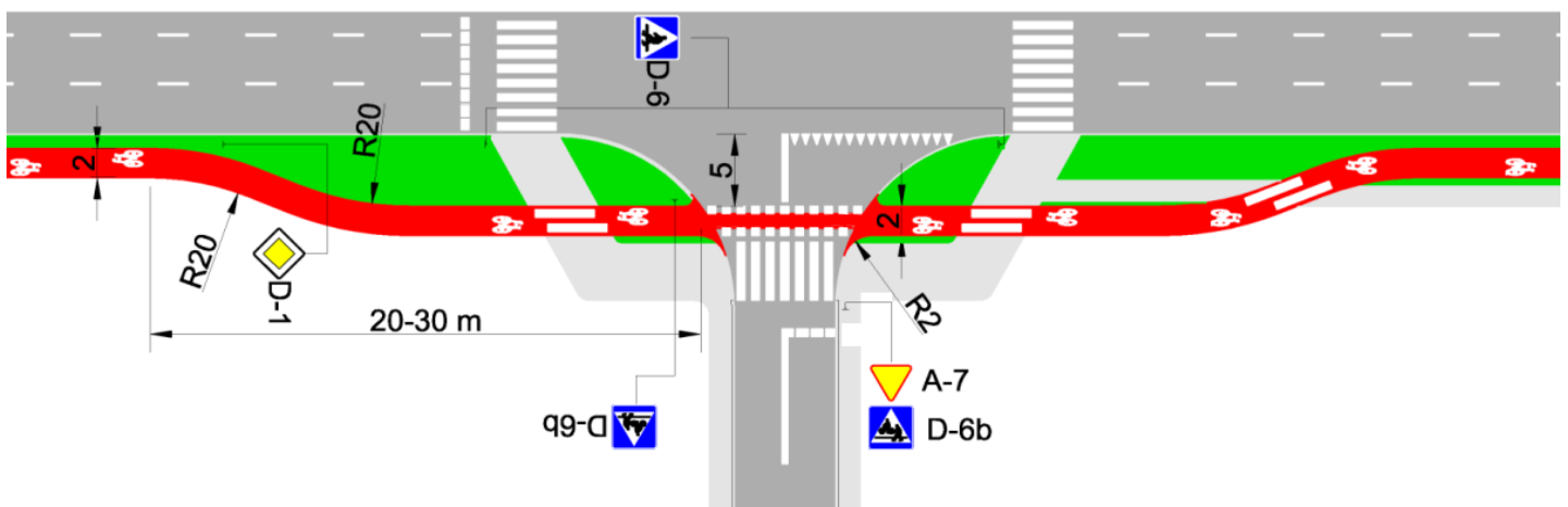
Rys. 21. Poprawny przebieg drogi dla rowerów w rejonie skrzyżowania: duże promienie łuków w dużej odległości od przejazdu dla rowerzystów. Zwracają uwagę wykrąglenia na styku drogi dla rowerów i jezdni ogólnodostępnej.
