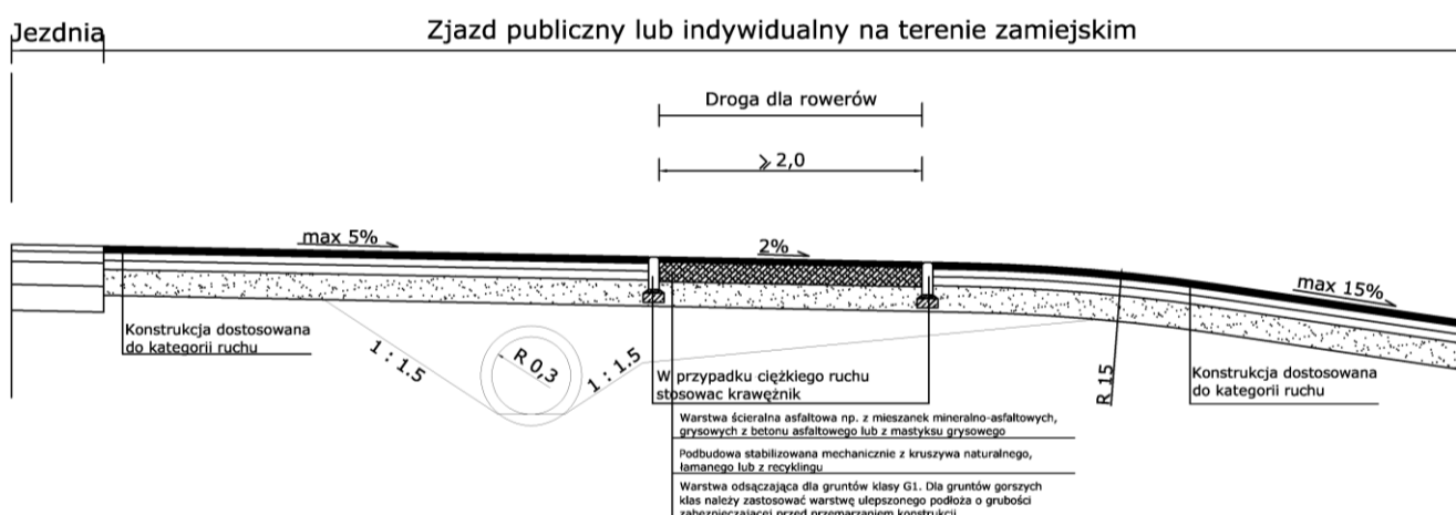
Rys. 12F. Przykład konstrukcji drogi dla rowerów na przecięciu zjazdu indywidualnego (droga zamiejska). Należy zwrócić uwagę, że sytuacja wysokościowa (spadki poprzeczne) może być zupełnie inna. Patrz też przykład na rys. 12G oraz rys. 13A.
