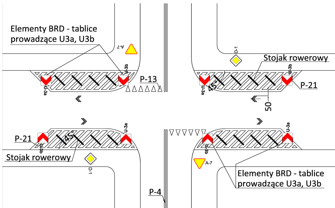
Rys. 26D. Przykładowa organizacja parkingów rowerowych w jezdni. Stojaki powinny być zabezpieczone z obu stron elementami małej architektury (betonowe donice itp.) oraz tablicami U-3. Lokalizacja parkingów na wlotach jezdni z pierwszeństwem poprawia pole widoczności na skrzyżowaniu. Dodatkowo możliwe jest stosowanie znaku D-18 „parking” z symbolem roweru.
