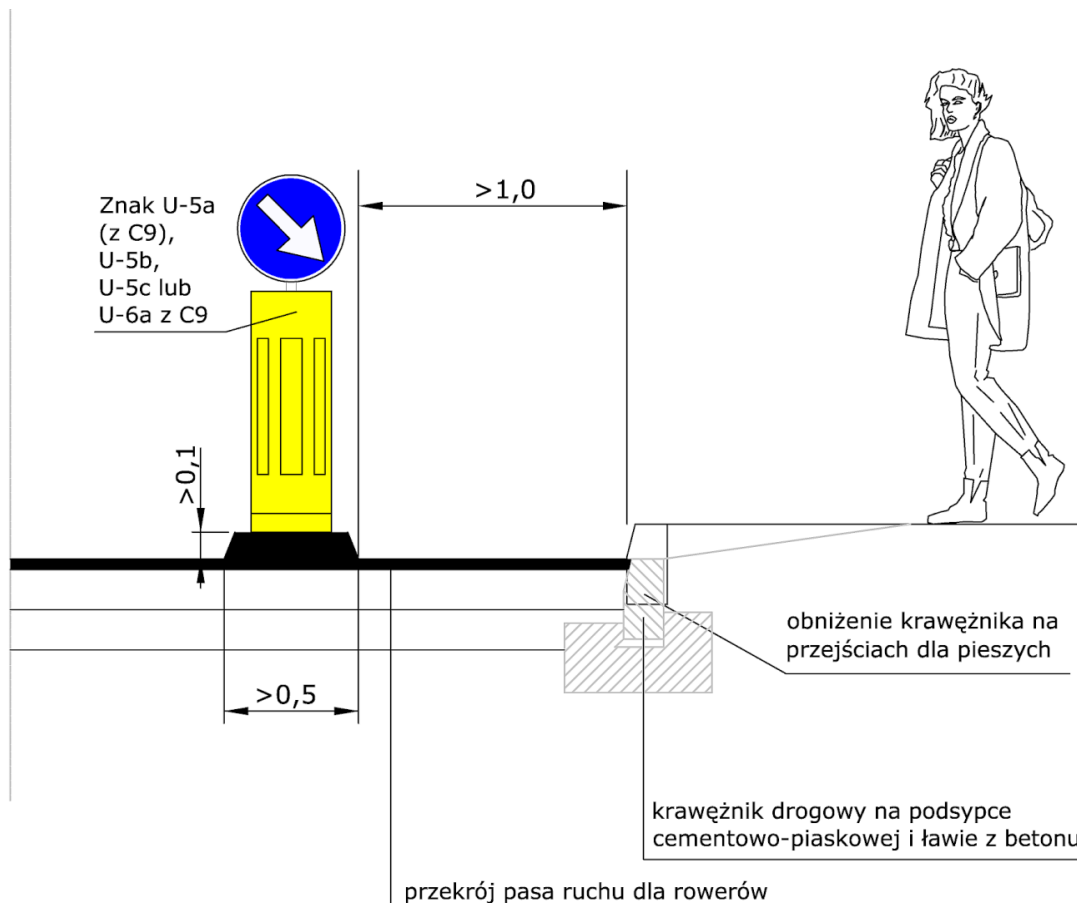
Rys. 11. Wyspa dzieląca ze słupkiem przeszkodowym U-5a/b/c (lub tablicą U-6a) oddzielająca pas ruchu dla rowerów (kontrapas) od pozostałej części jezdni. Widoczne dopuszczalne wyjątkowo zwężenie pasa ruchu dla rowerów do 1,0 m w poziomie niwelety.
