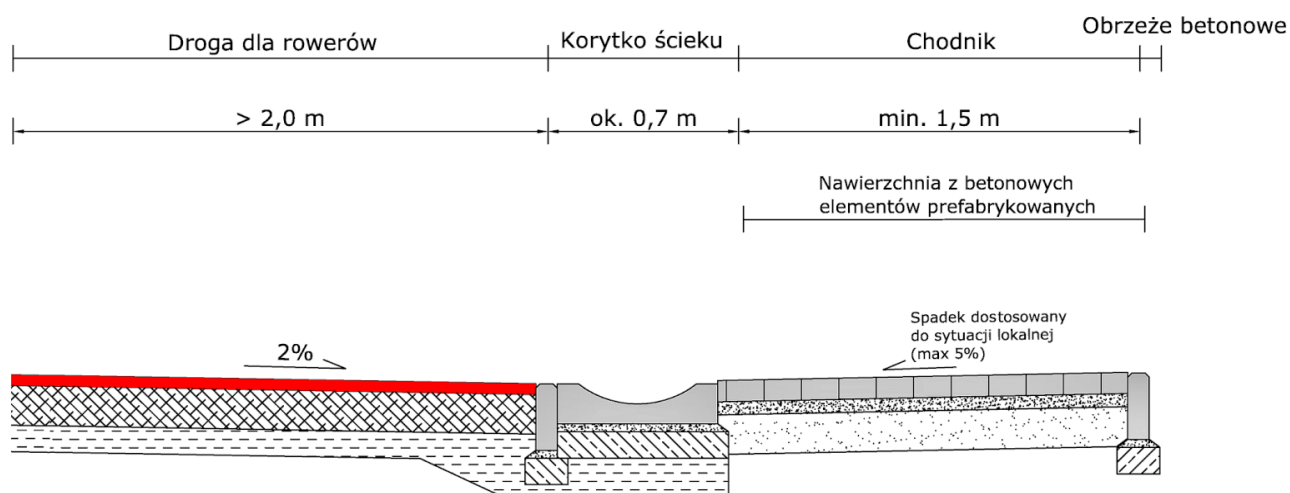
Rys. 12E. Przykład konstrukcji dwukierunkowej drogi dla rowerów oddzielonej od chodnika prefabrykowanym otwartym ściekiem korytkowym o przekroju wycinka koła.
