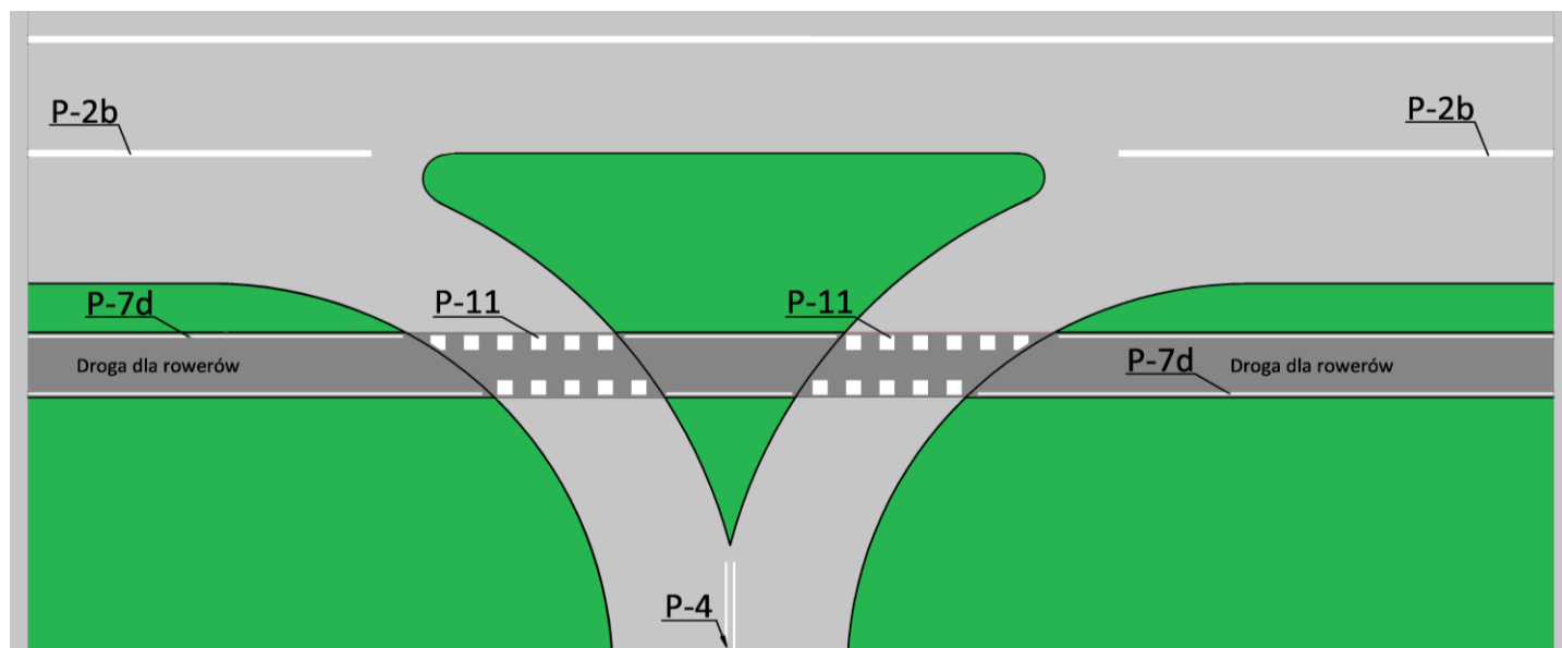
Rys. 12J. Zjazd publiczny w rzucie poziomym: należy zachować oś drogi dla rowerów równoległą do osi drogi głównej niezależnie od geometrii zjazdu
