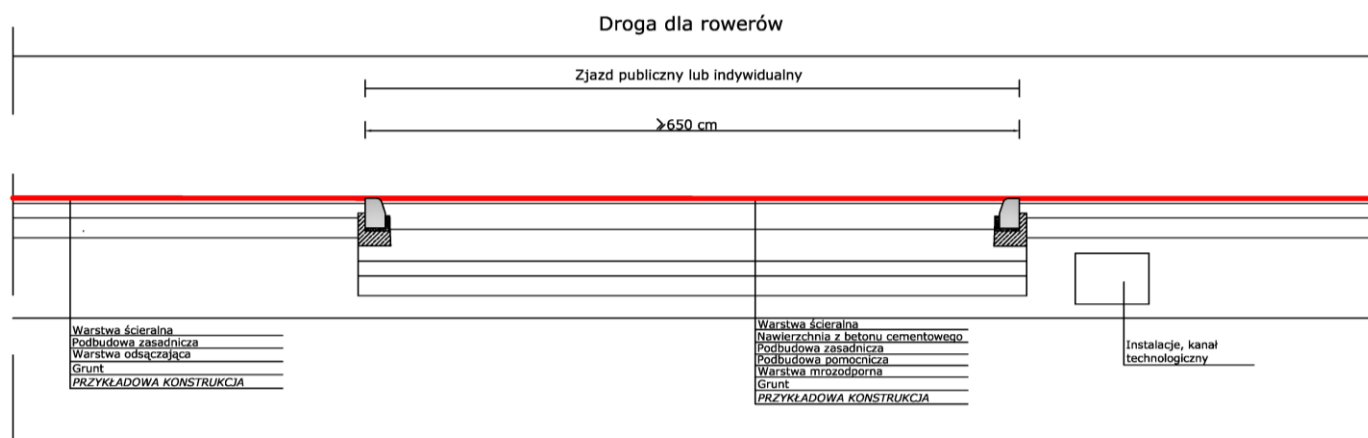
Rys. 12H. Przykład konstrukcji zjazdu publicznego lub indywidualnego – przekrój podłużny drogi dla rowerów (przekrój poprzeczny zjazdu). Zjazd ograniczony wtopionymi krawężnikami na ławie z betonu cementowego.
