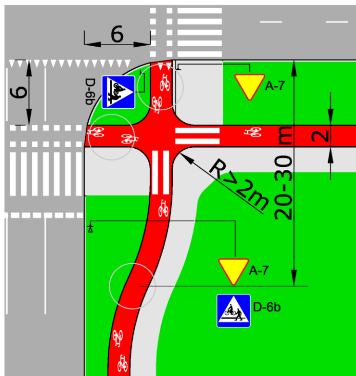
Rys. 22D. Przykładowy przebieg dróg dla rowerów w narożniku dużego skrzyżowania zwykłego z sygnalizacją świetlną. Zaznaczono obszary automatycznej (zdalnej) detekcji rowerzystów. Zwraca uwagę oznakowanie poziome i pionowe ustalające pierwszeństwo na przejazdach dla rowerzystów.
