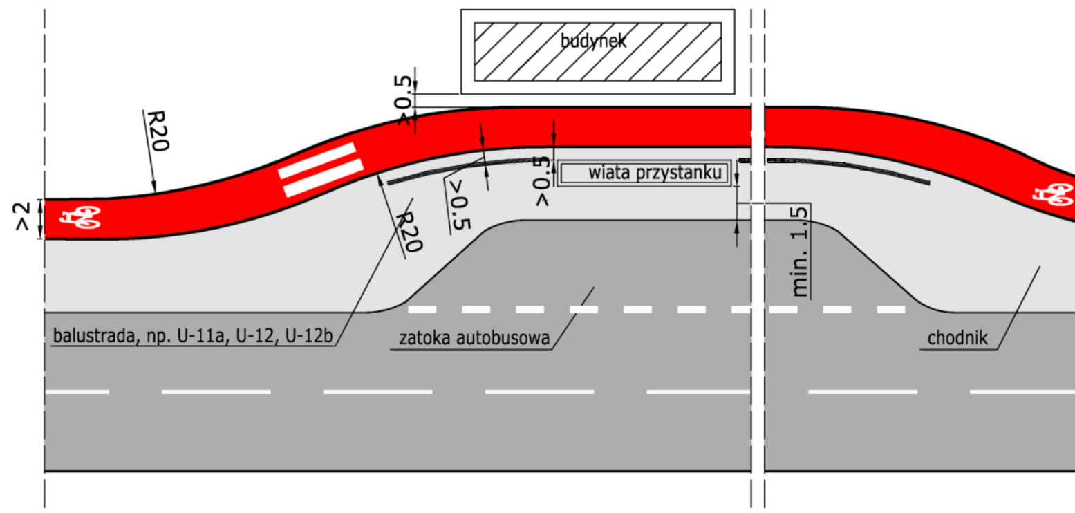
Rys. 16. Przykładowy przebieg drogi dla rowerów w rejonie przystanku autobusowego
