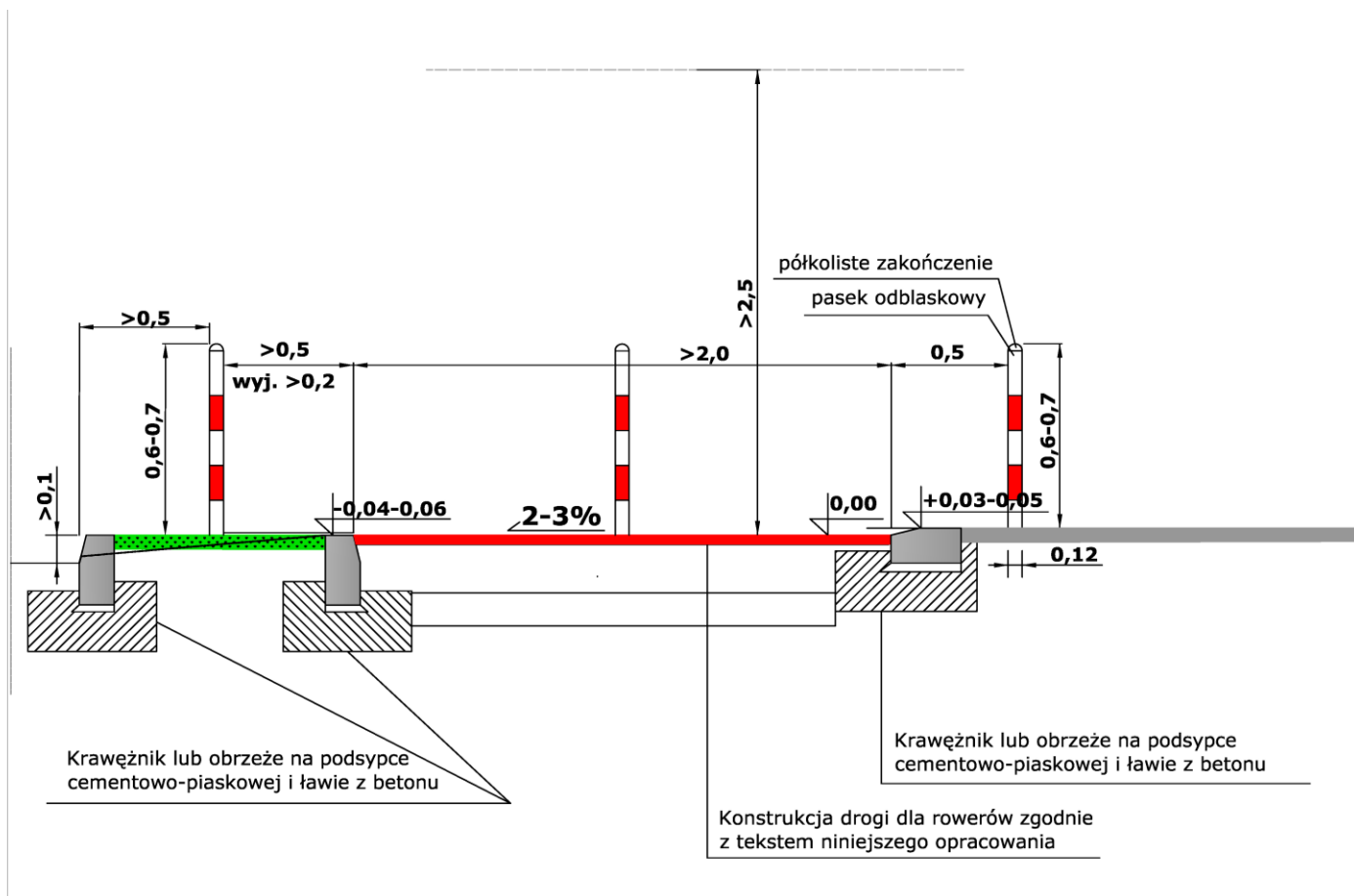
Rys. 12B. Inny przykład rozwiązania konstrukcyjnego drogi dla rowerów - przekrój poprzeczny dwukierunkowej drogi dla rowerów o nawierzchni bitumicznej, wariant zamknięty z obu stron krawężnikami drogowymi, w tym leżącym krawężnikiem drogowym (np. najazdowym) oddzielającym ją od przylegającego chodnika. Zastosowanie słupków U-12c jest opcjonalne, muszą one jednak znajdować się w odległości 0,5 m od krawędzi drogi dla rowerów (wyjątkowo 0,2 m) a środkowy – w osi dwukierunkowej drogi dla rowerów.
